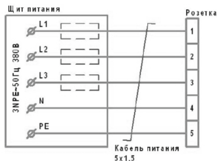
Рис. 5 Схема подключения розетки к стационарной сети
