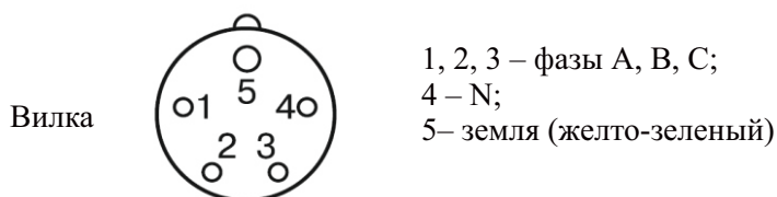
Рис. 4 Схема контактов на вилке
