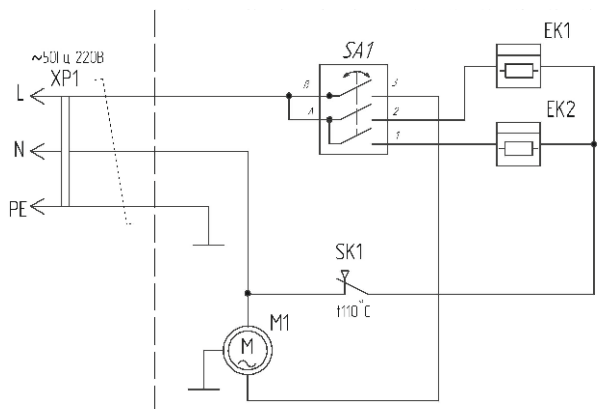
рис. 3 Схема электрическая.
